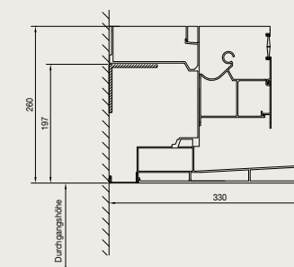
Pivot gevelmontage
