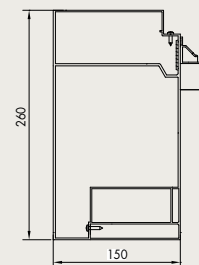
Span gevelmontage
