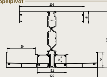
Koppelpivot
