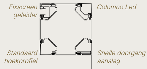
Kolom
